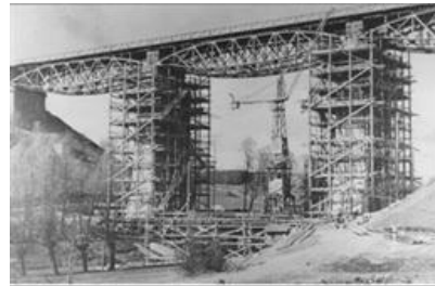
Emskirchner Brücke Umbau 1938 (Archiv HV)
